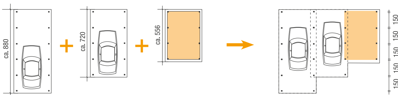
Sonderanfertigung, mit zwei versetzten Stellplätzen und seitlichem Geräteraum
