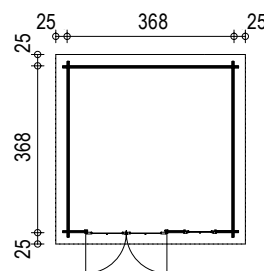
368 x 368 cm (baus. farbbeh.)
