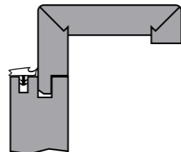
ZARGE MIT KLEINER RUNDKANTE, 60 MM BEKLEIDUNG FRAME WITH SMALL ROUNDED EDGE, 60 MM CASING
