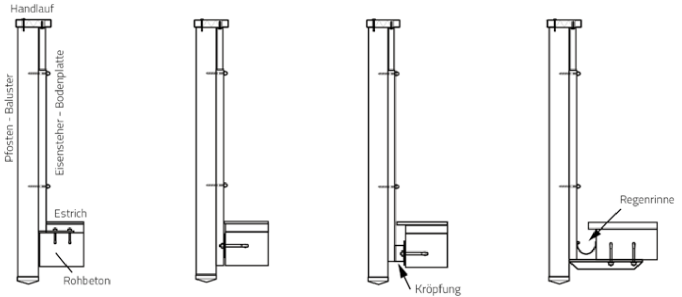
Eisensteher mit Bodenplatte zur Montage von oben auf die Betonplatte.
