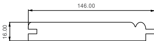
Altdeutsches Profil
