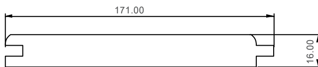
Rundfaseprofil
